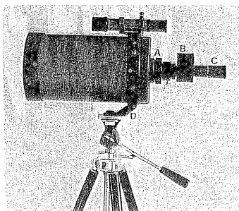
The Porro Prism (A) Visual back (B) Porro Prism (C) Ocular (D) C5 photo tripod adapter
